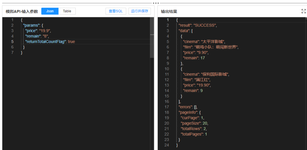
图 4-2 模拟 API
